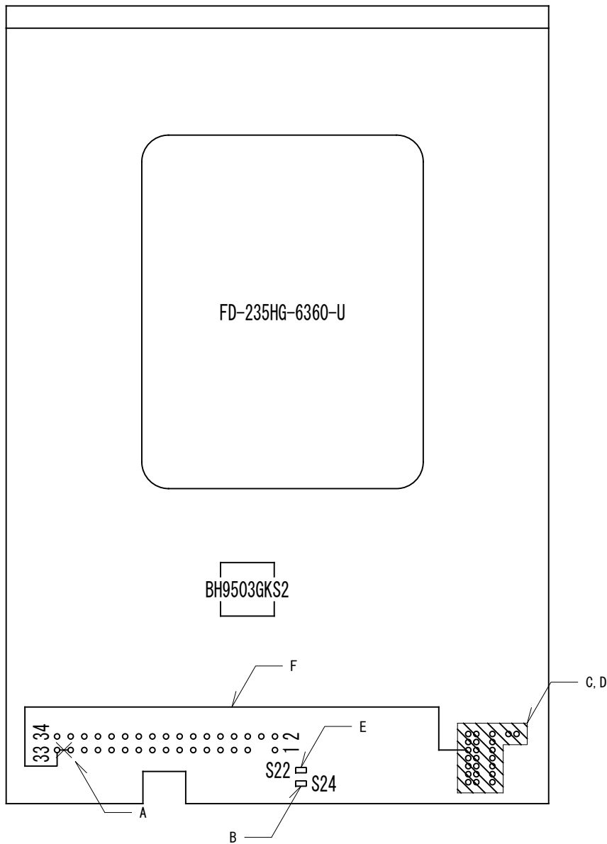
FDD基板 改造位置 プロット図 S=N/S
