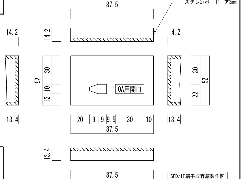
SPD/IF端子収容箱製作図 (Dreamcast用) S=1/2
